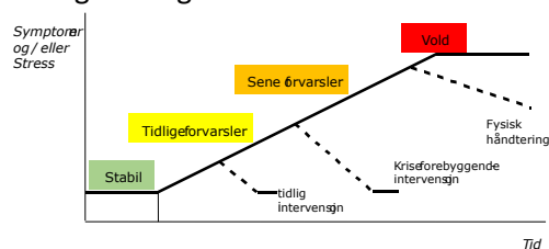
Fig. 1. Tilbakefallsprosessen
